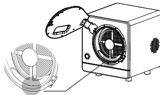
船錨型滾筒支架確實置入定位孔
